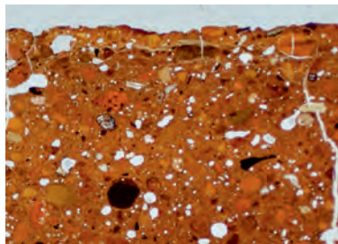
Dünnschliff eines historischen Verfumörtels
