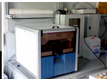
Gravisorp 120 zur Sorptionsanalyse von Baustoffen
