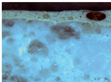
Schichtenaufbau einer Putz- und Anstrichprobe
